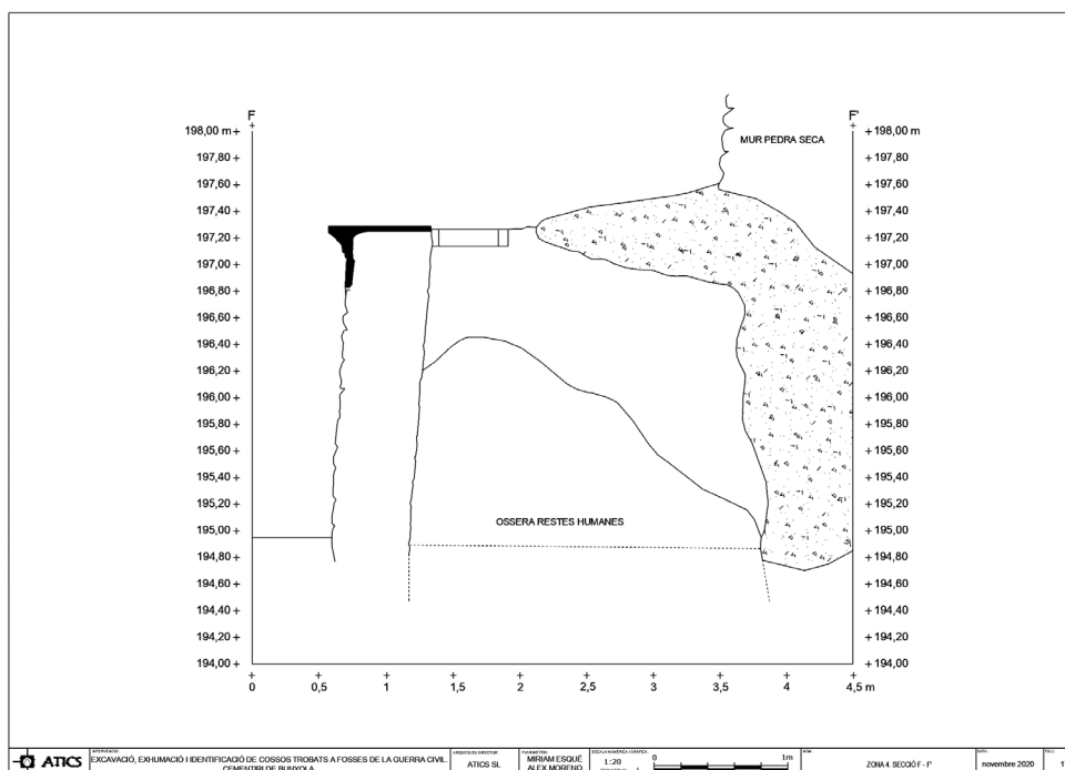
Figura 8. Secció de l'ossera de la zona 4.
