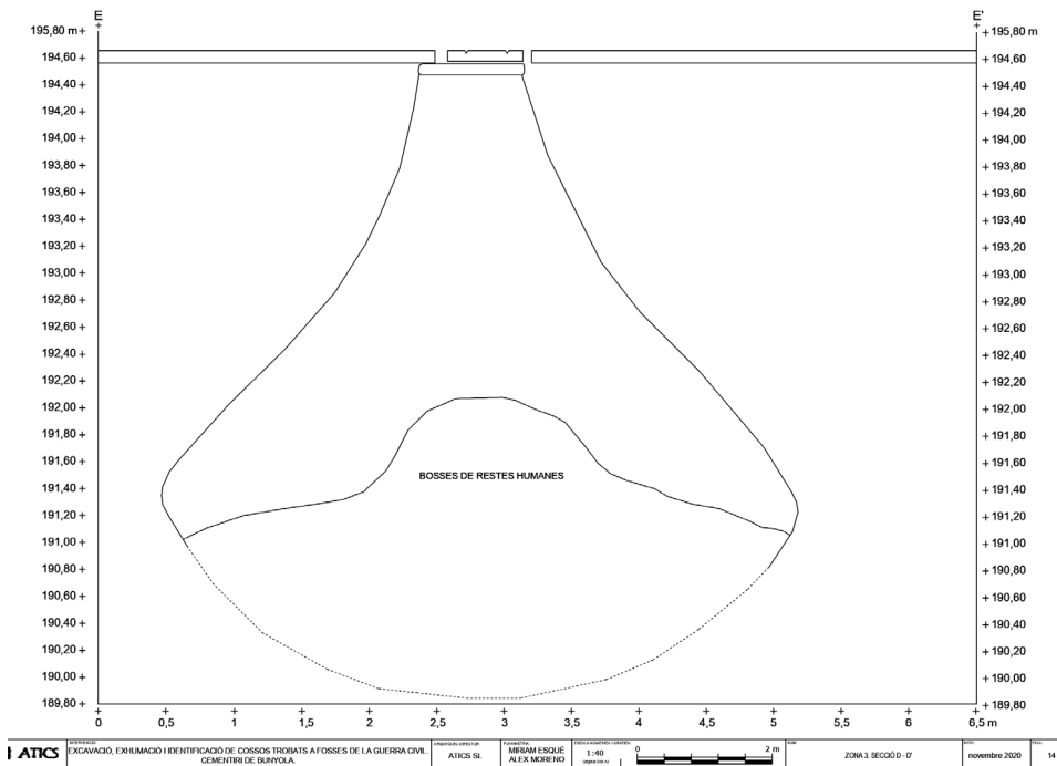
Figura 5. Secció de l'antic aljub reutilitzat com a ossera actual.
