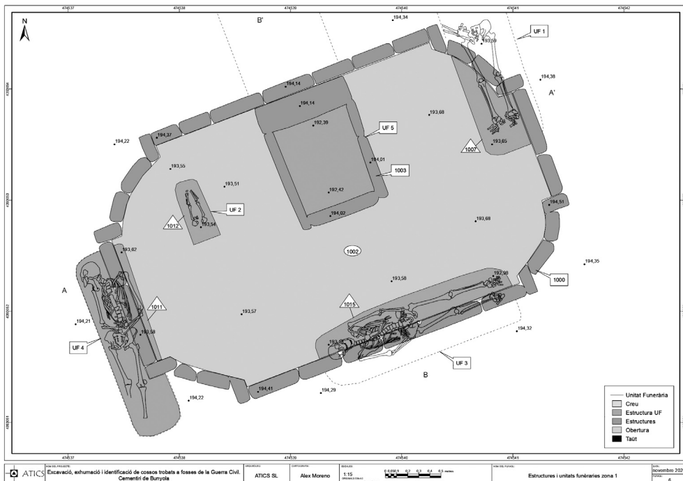
Figura 3. Zona 1 amb la indicació de les unitats funeràries excavades.
